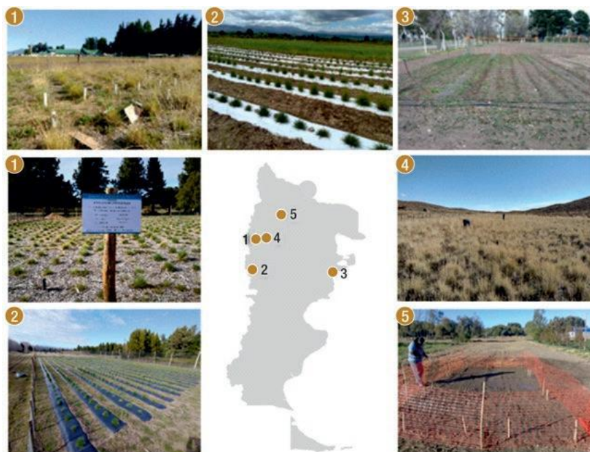
Figura 6. Imágenes de los ensayos de campo y parcelas demostrativas instalados con F. pallescens y su ubicación geográfica. 1: EEA Bariloche; 2: CEAT Trevelin; 3: EEA Chubut; 4: Pilcaniyeu (Parcela inscripta ante INASE); 5: Picún Leufú.
