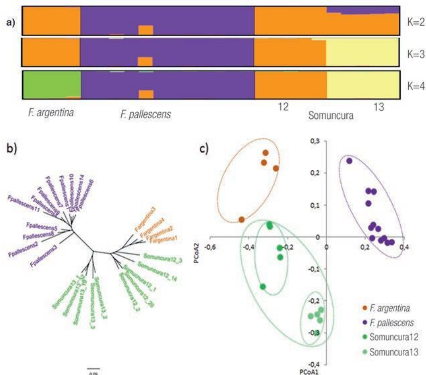
Figura 2. Caracterización genética de poblaciones de F. pallescens de Patagonia norte y comparación con la especie simpátrica F. argentina mediante marcadores microsatélites. Se destaca la diferencia genética de las poblaciones de la meseta de Somuncura. a) Análisis de estructuración genética entre poblaciones (STRUCTURE); b) Árbol filogenético (radial neighbour-joining); c) Análisis de coordenadas principales, ambos a partir de la distancia genética de Bruvo para organismos poliploides. Se distinguen cuatro grupos: F. pallescens (violeta), F. argentina (naranja) y las dos poblaciones de la Meseta de Somuncura (verde claro y oscuro) (modificado de López et al. , 2018)
