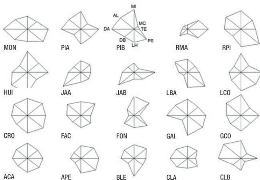
Figura 5. Gráfico de estrella en donde se observa de manera resumida la variabilidad en los diferentes caracteres medidos entre las poblaciones estudiadas. MI, número medio de macollos registrados en los primeros 90 días posgerminación en invernáculo. MC, número medio de macollos registrados en el primer período de floración a campo. TE, tiempo de emergencia total. LH, longitud de hoja en los primeros 90 días posgerminación en invernáculo. DB, diámetro de la corona de las plantas de 2 años. DA, diámetro aéreo de las plantas de 2 años. AL, altura modal de las plantas de 2 años. Poblaciones evaluadas: ACA, HUI, CLA, CLB (Neuquén), PIA, PIB, JAA, JAB (Río Negro), MON, APE, CRO, GCO, RPI, FON, FAC, RMA (Chubut), LBA, GAI, BLE, LCO (Santa Cruz.)
